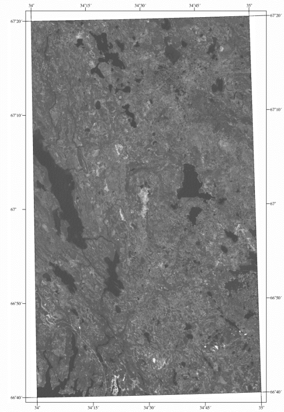
ДИСТАНЦИОННАЯ ОСНОВА 3 канал (0,63-0,69 мкм) KC LANDSAT
