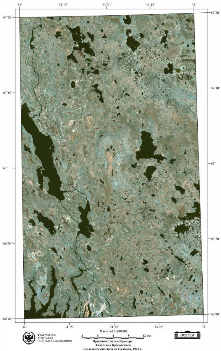
ДИСТАНЦИОННАЯ ОСНОВА Цветовая композиция RGB 3-го, 2-го и 1-го каналов, объединенных с панхроматическим каналом Q-36-XI
