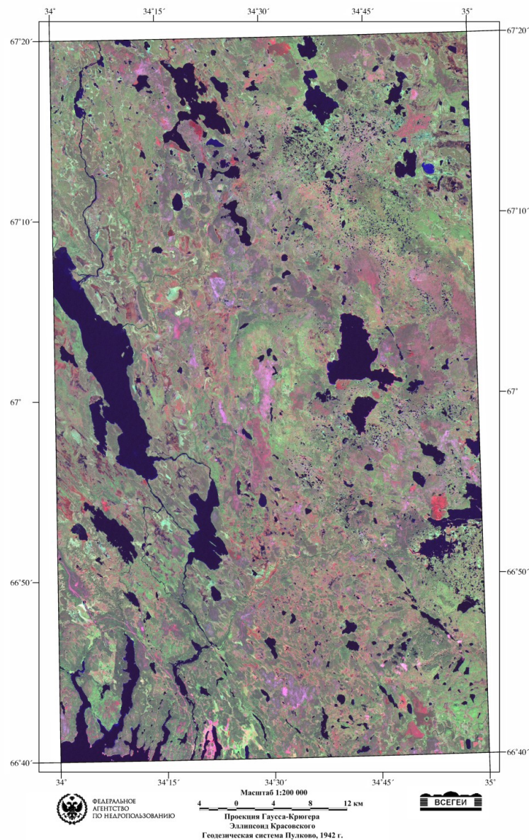
ДИСТАНЦИОННАЯ ОСНОВА Цветовая композиция RGB 7-го, 4-го и 2-го каналов, объединенных с панхроматическим каналом Q-36-XI
